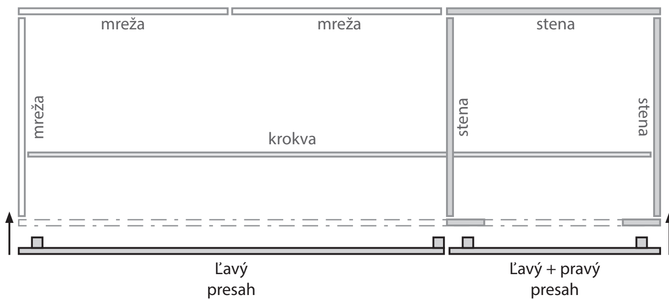
Umiestnenie čelových panelov – pôdorys
